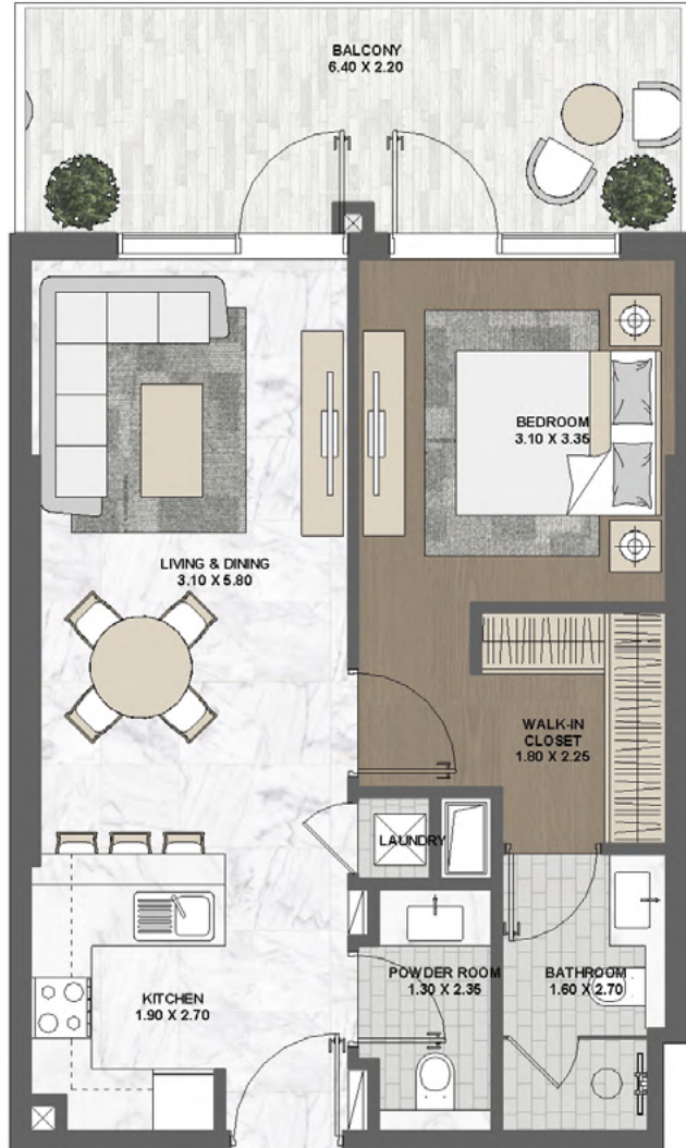
1BR - 01
