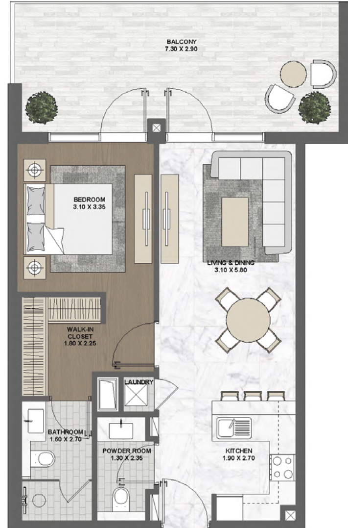
1BR - 02
