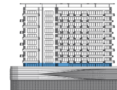
ELEVATION B
